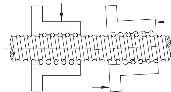
Fig 1.11.1 Offset Load
